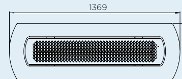
MARCO DE MONTAJE EMPOTRADO EN EL TECHO 2000 W Y 4000 W
