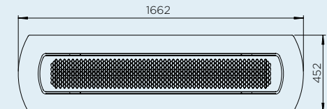
MARCO DE MONTAJE EMPOTRADO EN EL TECHO 3000 W Y 6000 W
